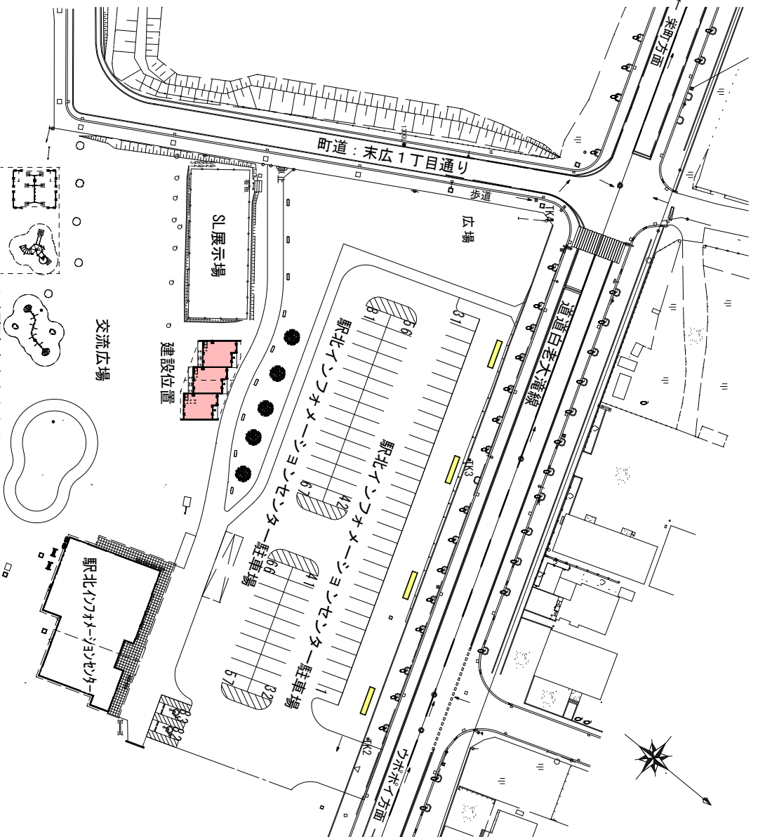
配置図 1 : 500
